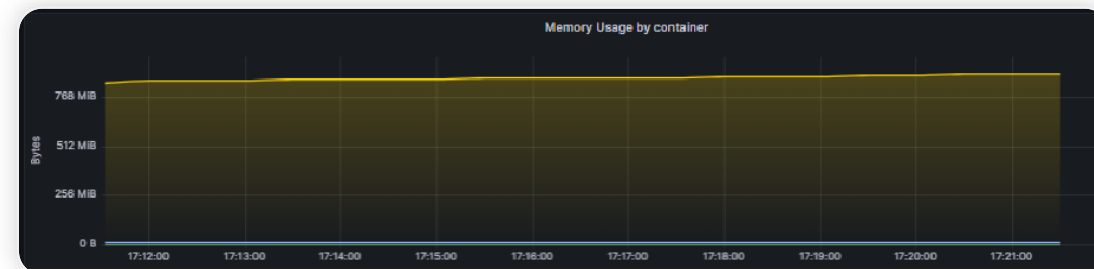
Утилизация ОЗУ
