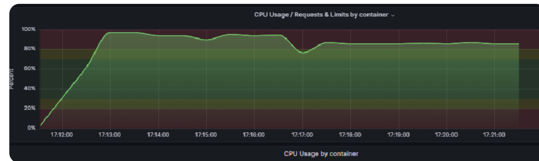
Утилизация ЦПУ
